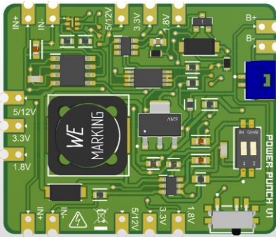
Top Layer
